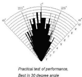
Рис 78. Диаграмма направленности сонара HC-SR04
